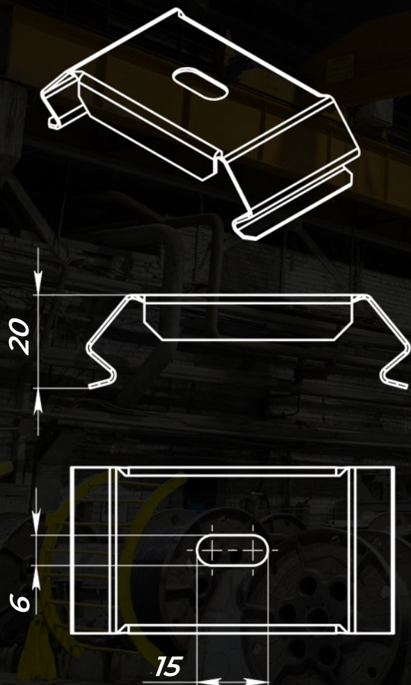
Металлическая клипса для светильника
